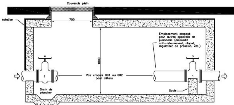
COUPE A-A (Aucune échelle)
